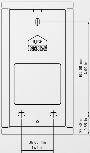
Gehäuseinnenseite
